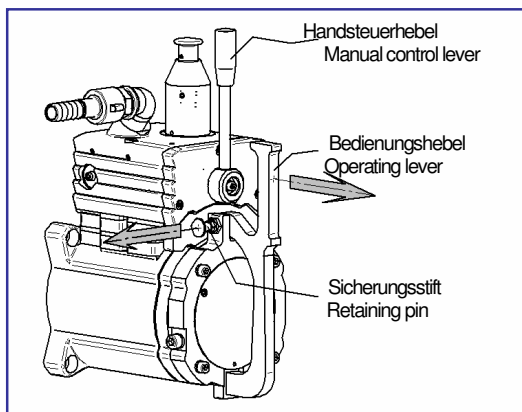
Not-Senk-Einrichtung bei JDN-Drahtseilwinden
