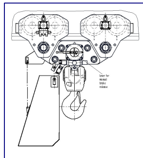
Druckluft-Kettenzug / Air Chain Hoist
